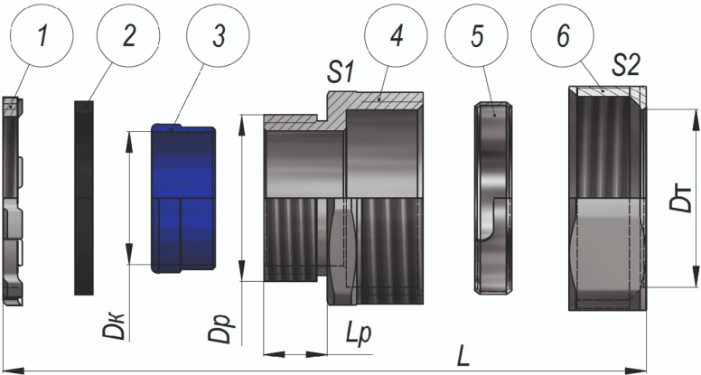
Рисунок 2 - Муфта вводная ATK. Основные технические данные.
