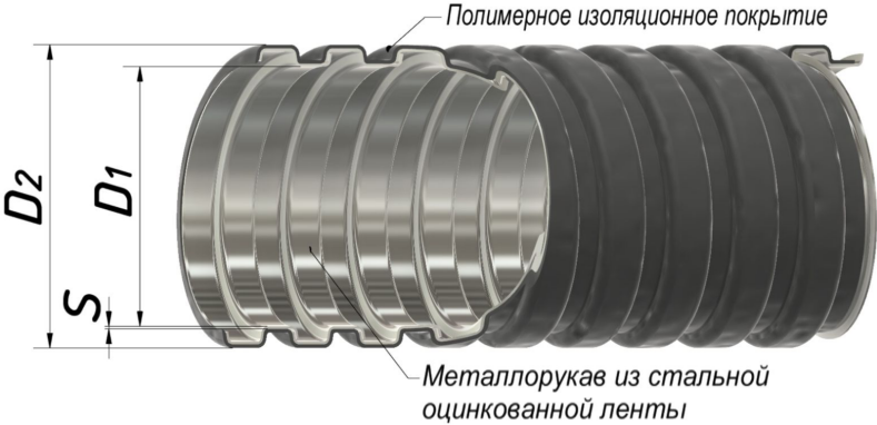
Рисунок 1. Металлорукав типа РЗ-ЦПнг
