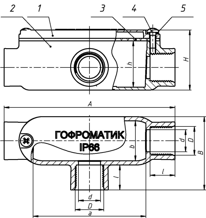
Рисунок 1 - Коробка алюминиевая Т-образная
