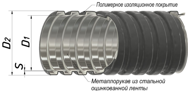
Рисунок 1. Металлорукав типа РЗ-ЦП нг-LS с протяжкой
