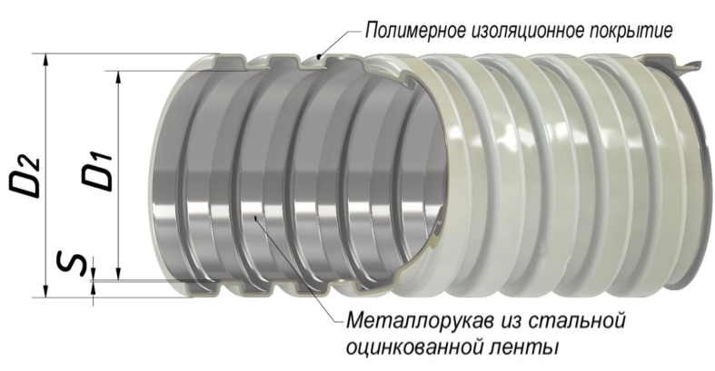
Рисунок 1. Металлорукав типа РЗ-ЦПнг серый
