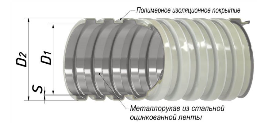
Рисунок 1. Металлорукав типа РЗ-ЦПнг серый
